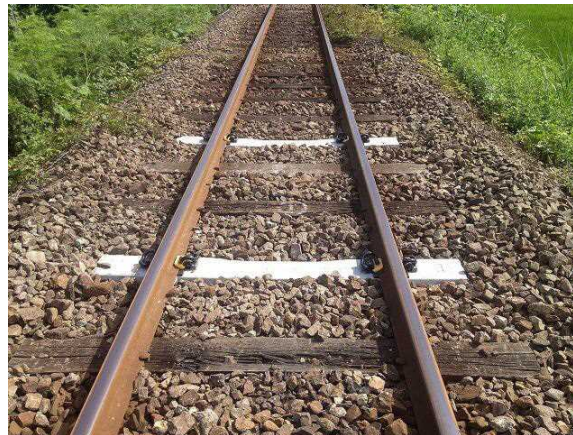
マクラギ交換 (秋田内陸線)
